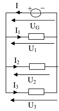
Circuit n°4
